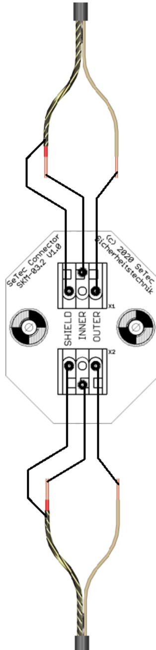
Abbildung 10 Anschluss Verbindungseinheit SKM-03.2
