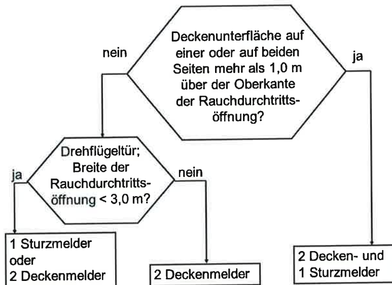
Bild 3: Entscheidungsdiagramm
