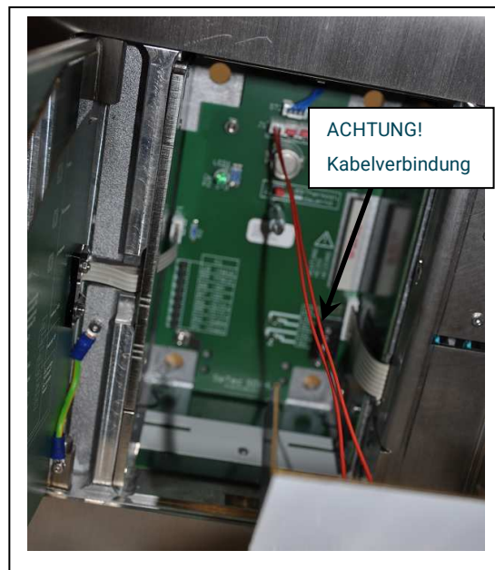
Kabelverbindung zwischen Konsole und Platine
